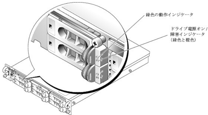
図 1-2 SCSI ハードドライブインジケータ
