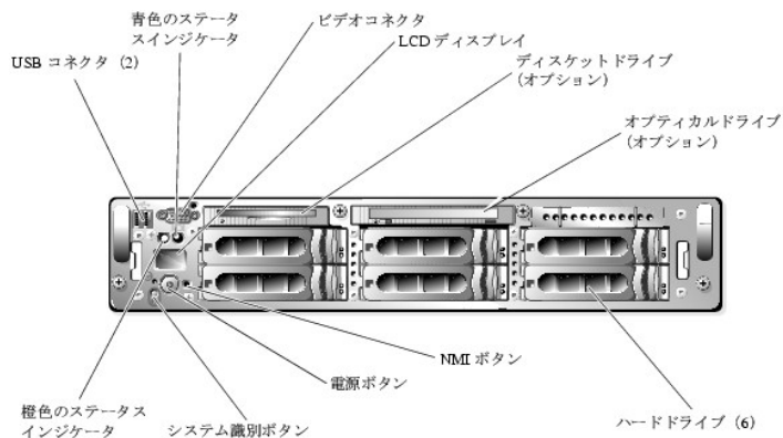
図 1-1 正面パネルの機能およびインジケータ
