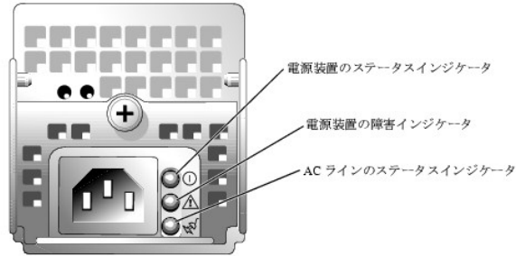
図1-4 冗長電源装置のインジケータ
